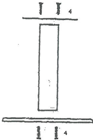
Montaje de la base : con 4+4 tornillos largos Assembly of the base : with 4+4 long screws
